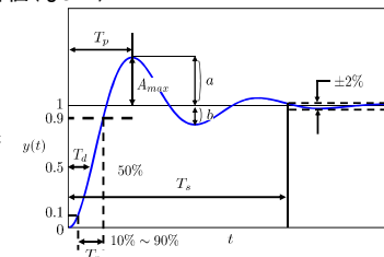
図3.10 過渡応答と諸特性値
