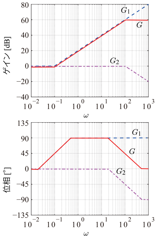
図 1: ボード線図
